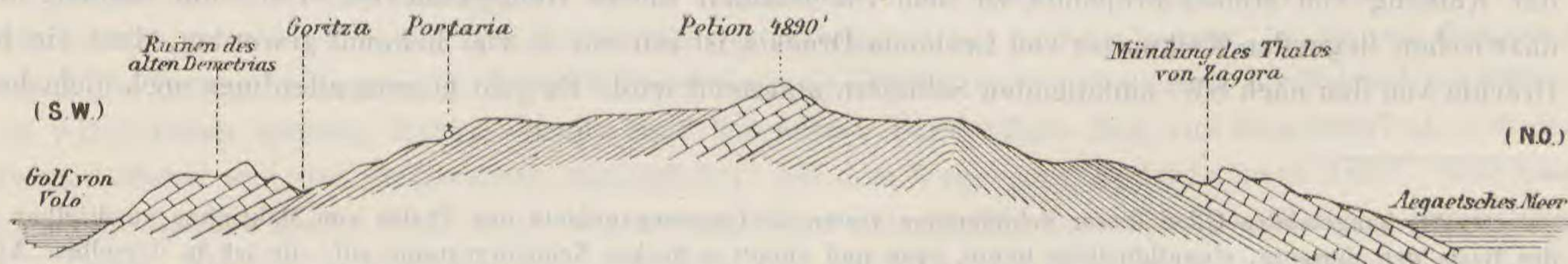
Fig. 2. Idealer Durchschnitt durch den Gebirgsstock des Pelion.
